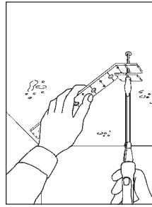
Deckenabhängler/Lochband ansetzen und abknicken
