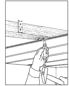
Tragfette ist montiert, Paneel wird angebracht
