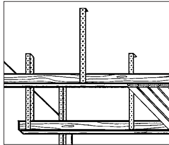
Deckenabhängung mit Lochbändern
