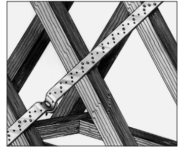
Aussteifung der Dachkonstruktion
